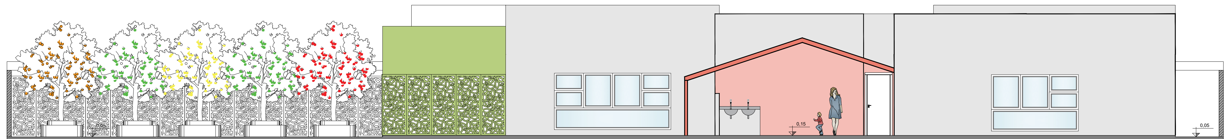
5 FACHADA POSTERIOR ESC. 1/75
