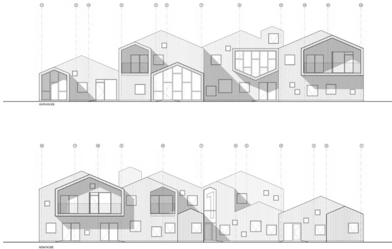
FACHADA FRONTAL E POSTERIOR
